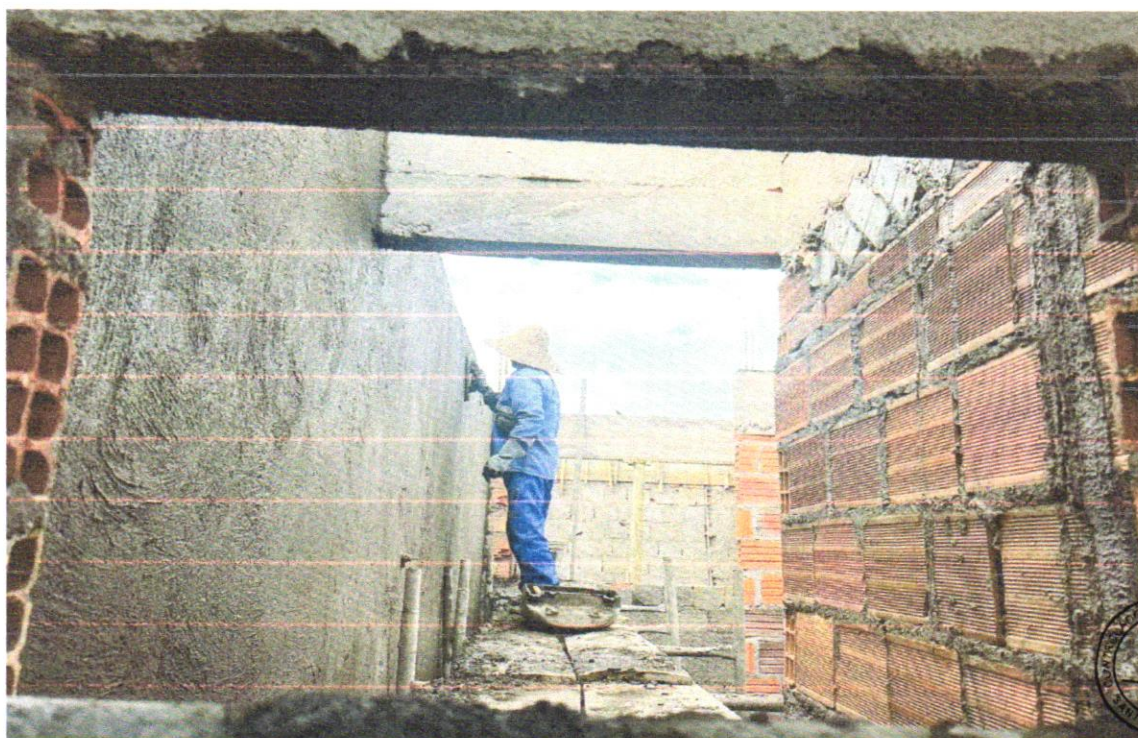
FOTO 26 – Reboco para paredes internas, externas, pórticos, vigas, traço 1:4,5 - espessura 0,5 cm
