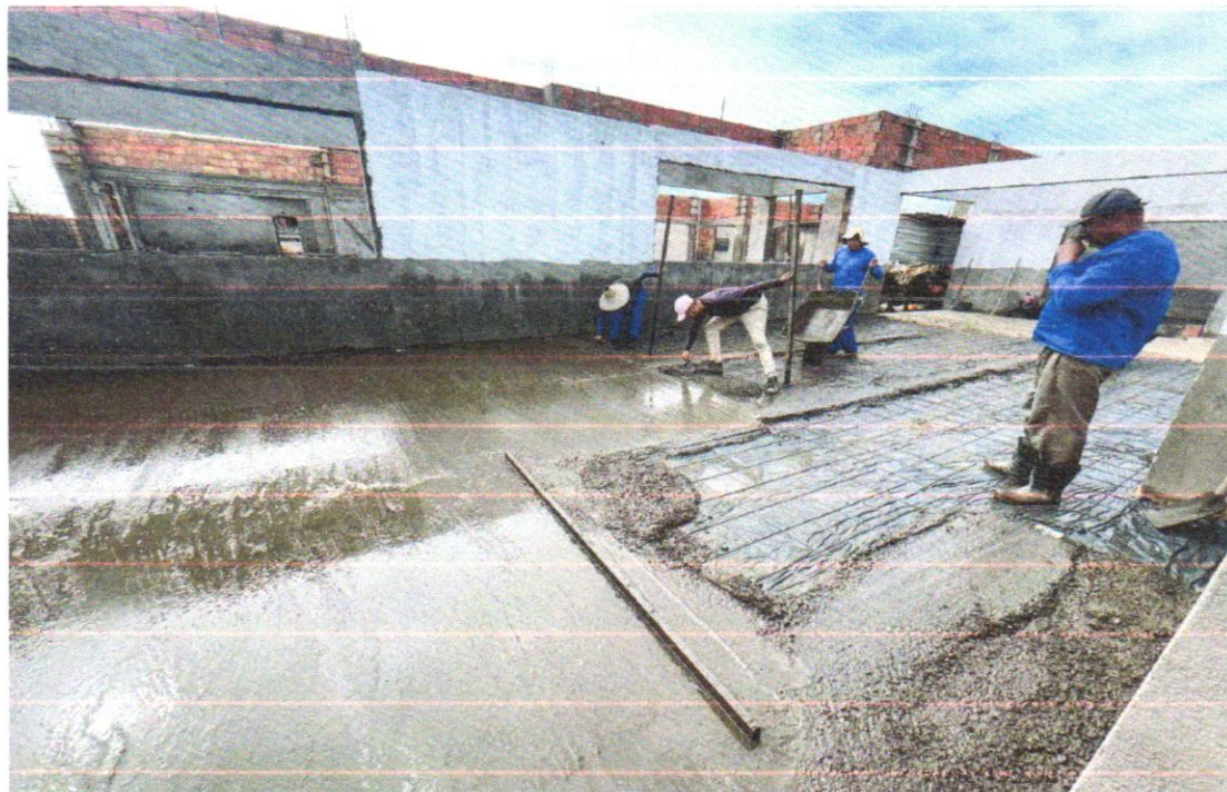
FOTO 50 – Contrapiso de concreto não-estrutural, espessura 3cm e preparo mecânico
